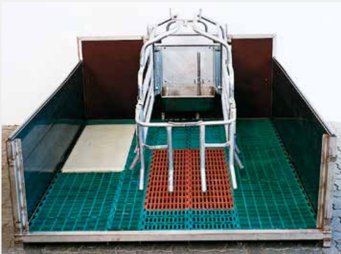
mit Kunststoffrost, Heizplatte für Ferkel und Gussrost unter der Sau
